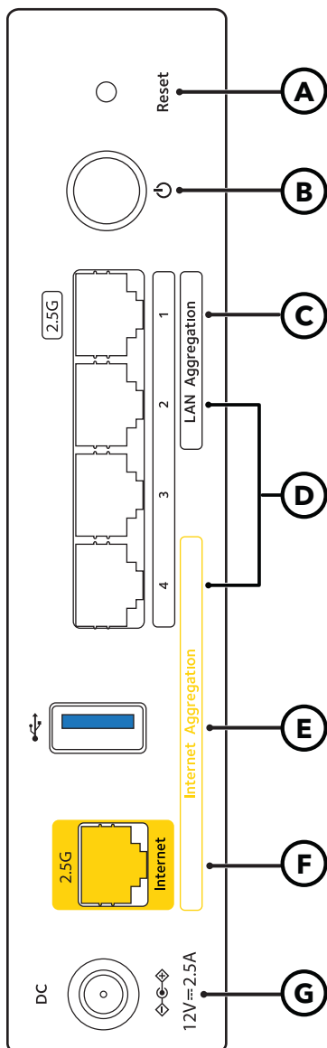
Illustration 3 : Panneau arrière
